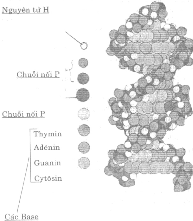
Mô hình ADN - theo E. Harbers (Trích trong Die Nuclein - säuren - 1964)
