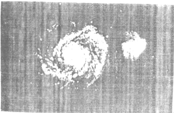
Trích sách: Welt-Erde-Mensch (Spiralnebel im Sternbild der Jagdhunde)S.51. (Tinh vân hình xoáy ốc của chòm sao “chó săn”)
